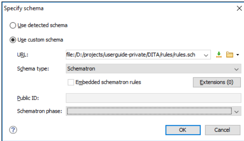
Figure 162: Specify Schema Dialog Box
