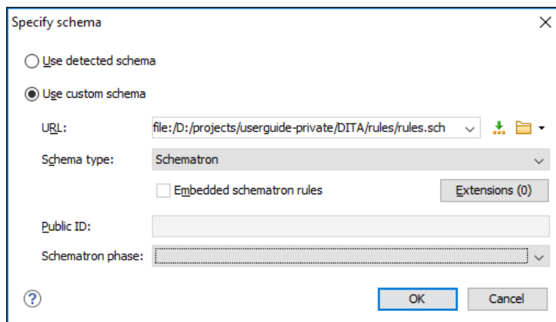
Figure 113: Specify Schema Dialog Box
